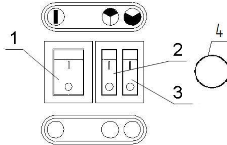
Рис. 1 Кнопки управления.
