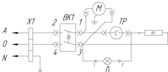
Принципиальная электрическая схема
