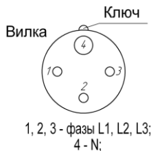
Рис.3 - Схема контактов на вилке
