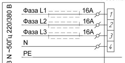
Рис.2 - Схема подключения розетки к стационарной электросети
