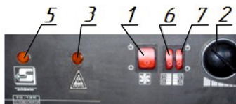
Панель управления ТВ-9К...24К
