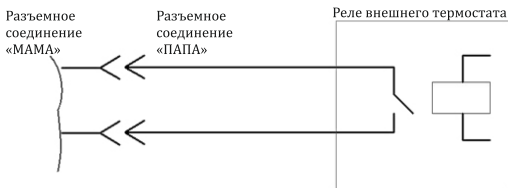
Рис. 8 Схема подключения ЭВП к внешнему термостату
