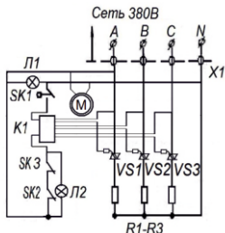
ЭВП-9; 12; 15; 18
